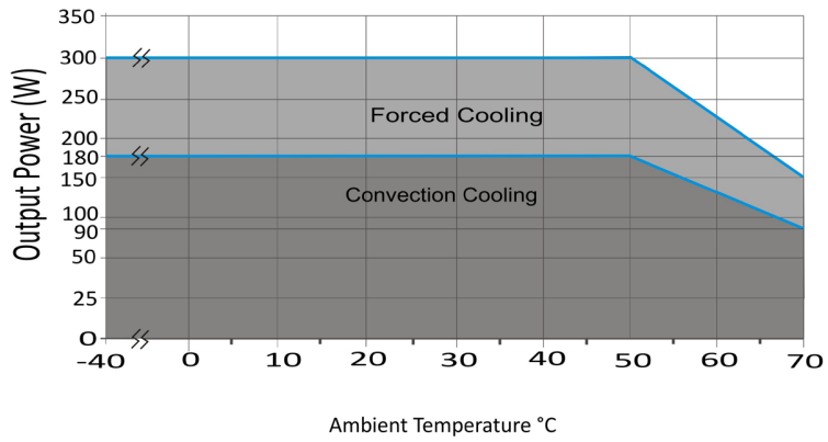
15V Output
